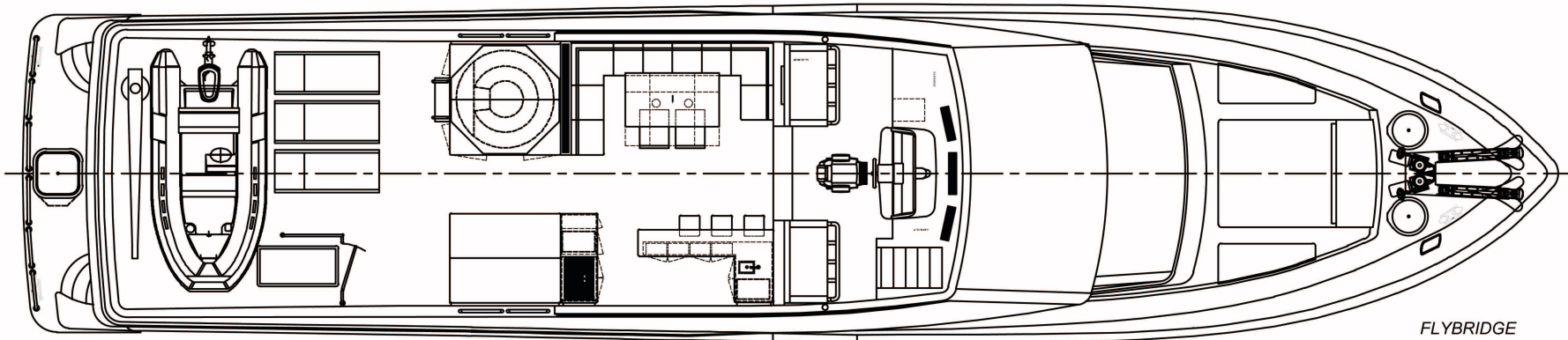
FLYBRIDGE
